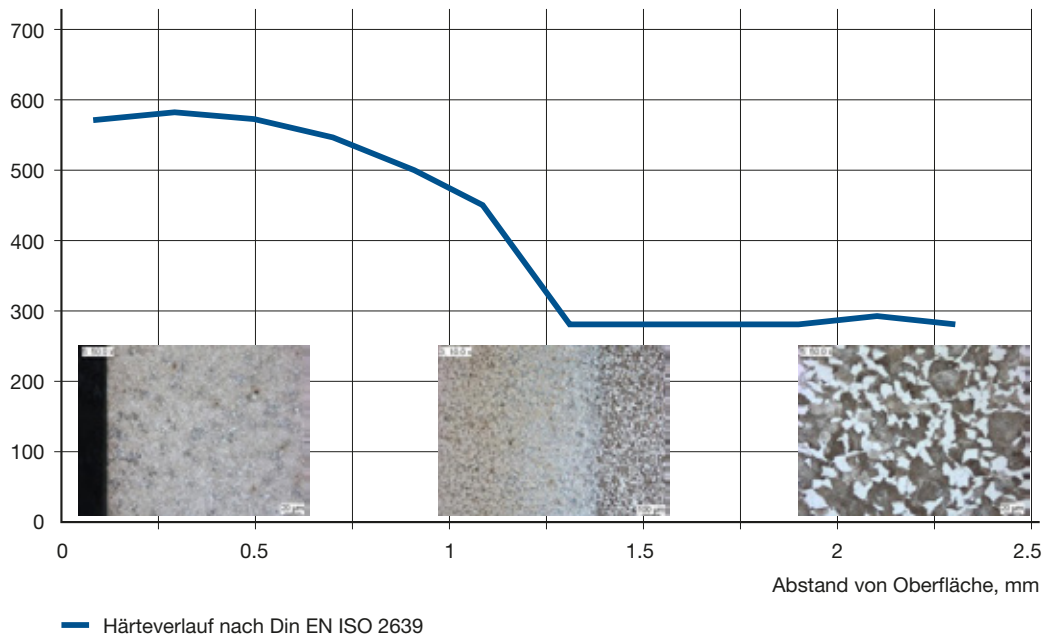
Härte HV10
