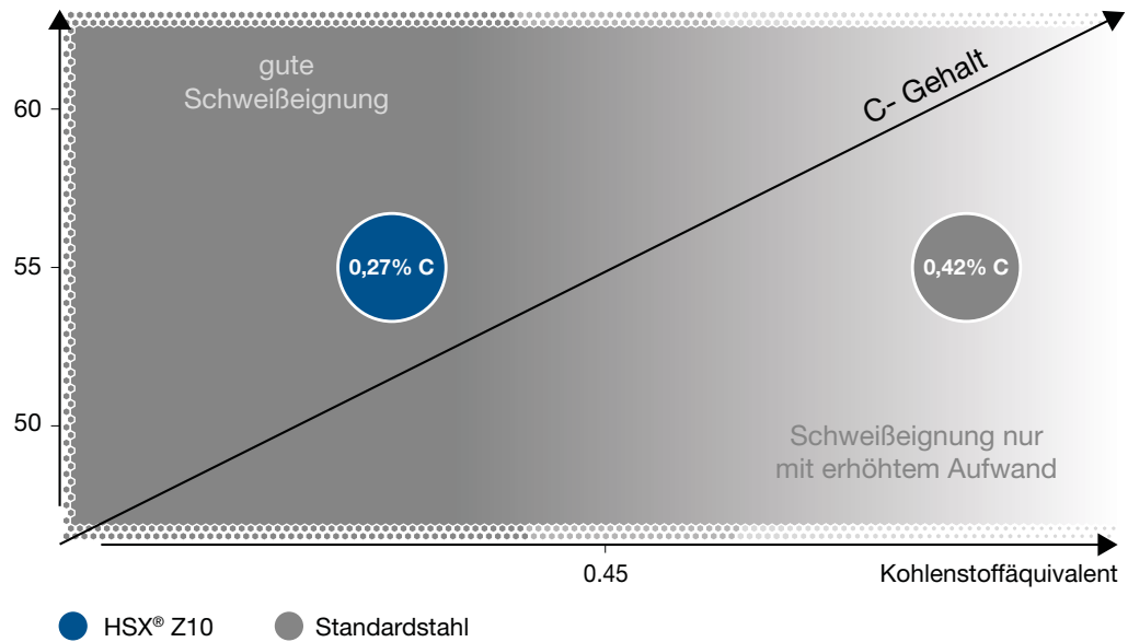
Oberflächenhärte in HRC nach Induktivhärten
